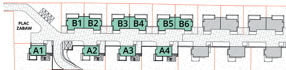
PLAN OSIEDLA
